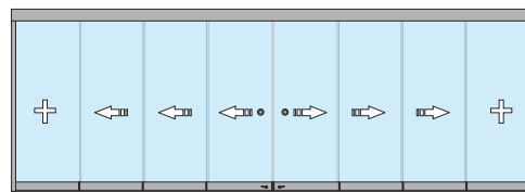
8 ante - 4 binari
